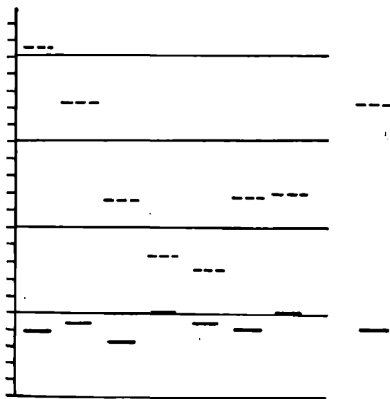
Обр. 14. а – стратиграфия на пластове в сондажа от 1977/78 г. на с. м. до с. Дядово, по Р. Катинчаров и др.; б – нива на средновековните ями, по Б. Борисов. Апендикс
